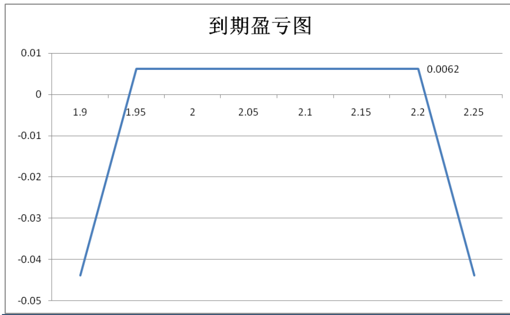
图 11：卖出宽跨式组合到期盈亏图
