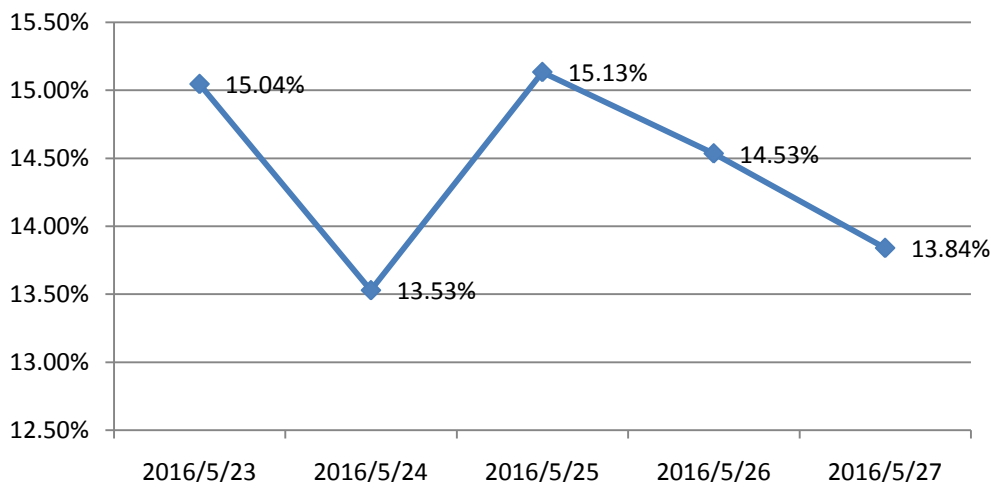
图 5: 上证 50ETF 期权综合隐含波动率一周走势图
