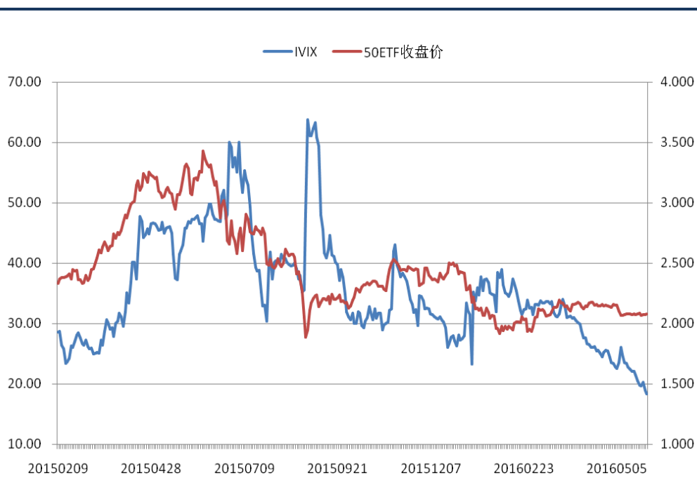
图 8：iVIX 指数走势图
