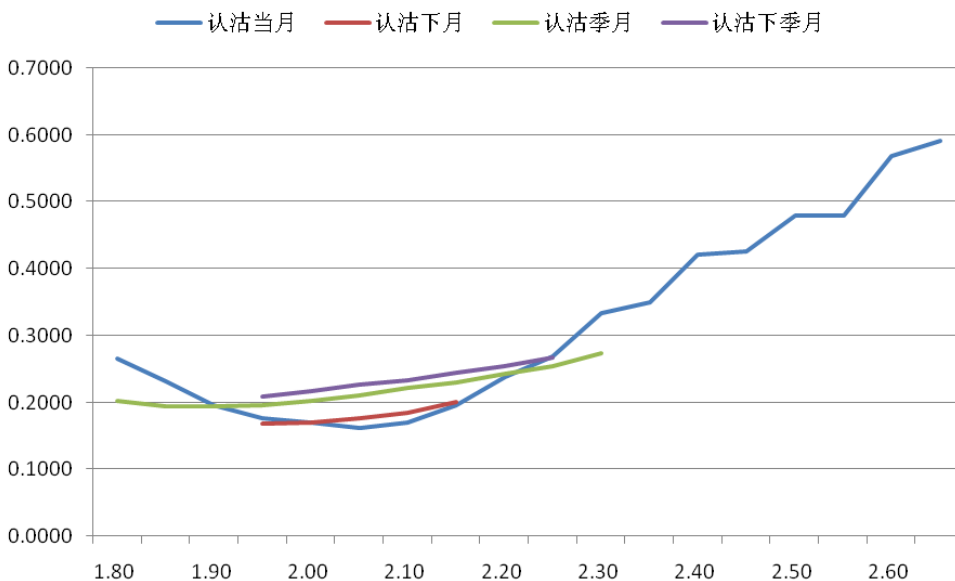
图 10：认沽期权隐含波动率微笑曲线（2016 年 5 月 27 日）
